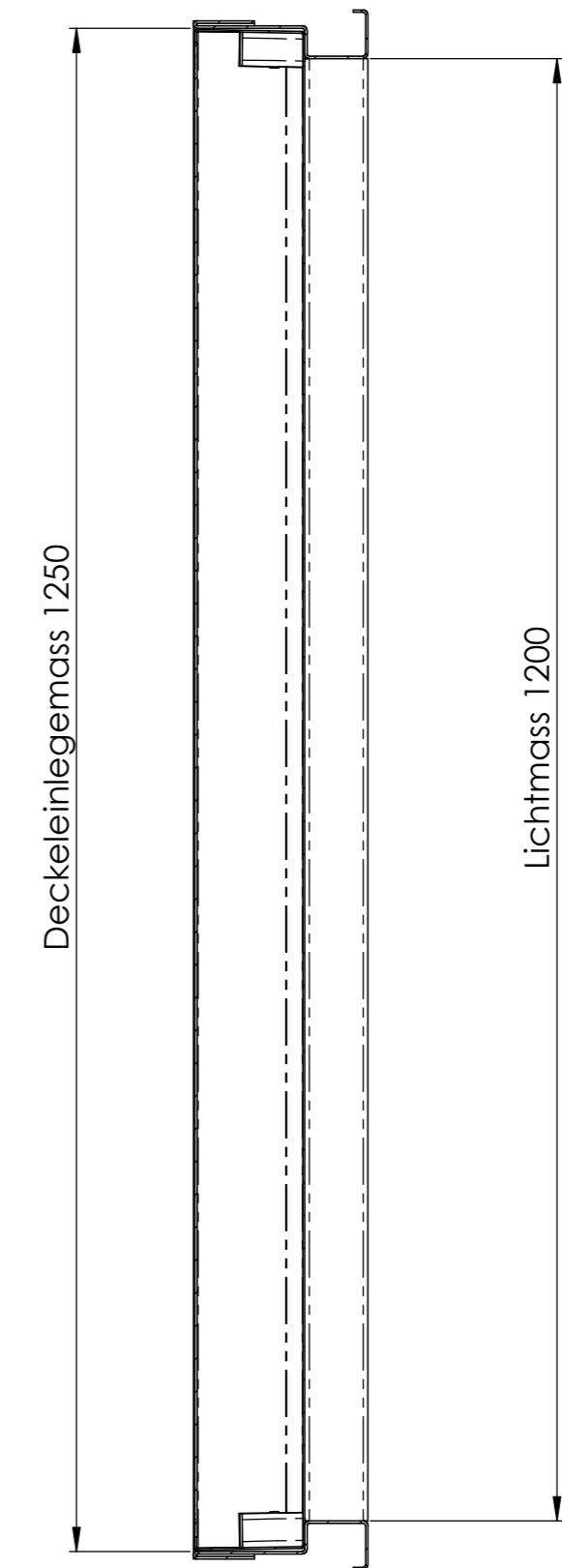
SCHNITT B-B MABSTAB 1 : 6
