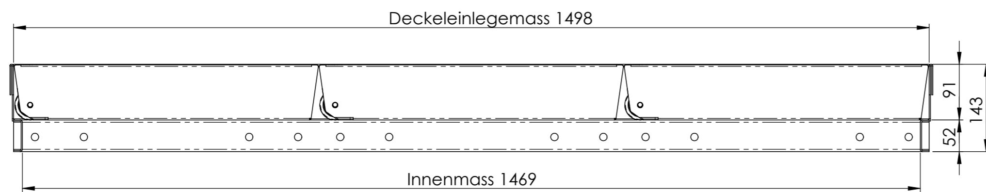
SCHNITT C-C MABSTAB 1 : 6
